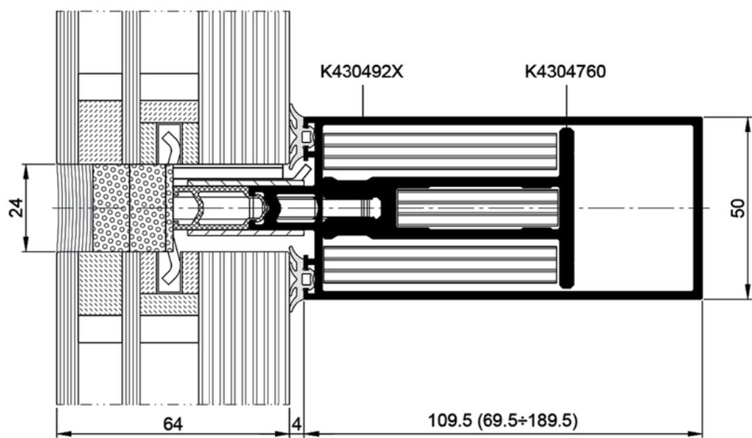
Przekrój przez rygiel EI60
