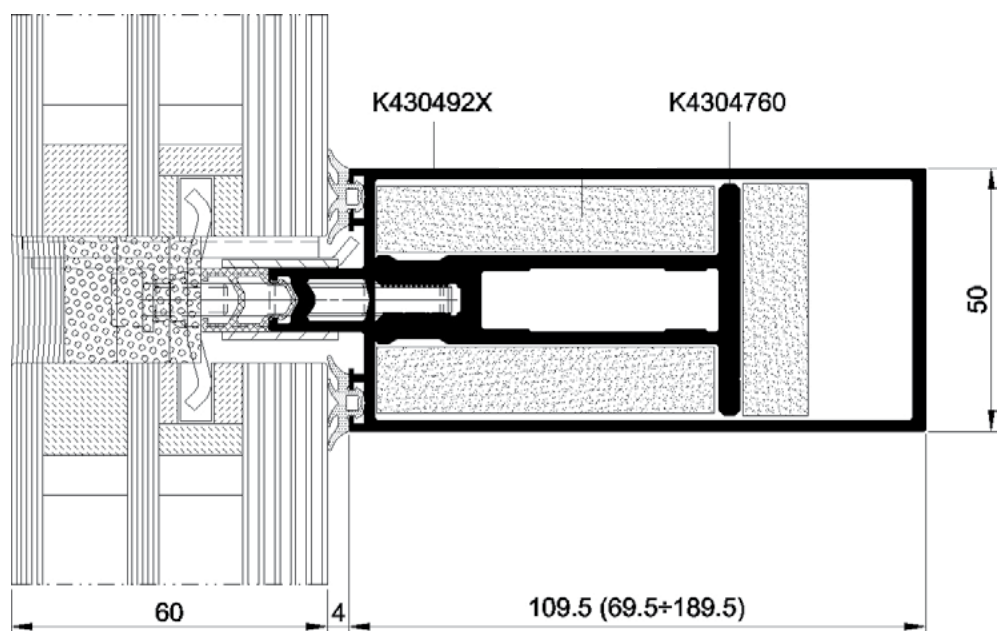
Przekrój przez rygiel EI30
