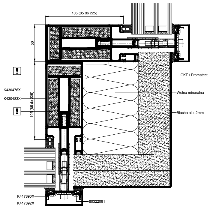
Przekrój przez słup 90o EI 30
